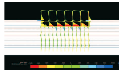
地盤と構造物の連成解析例(有効応力解析)
