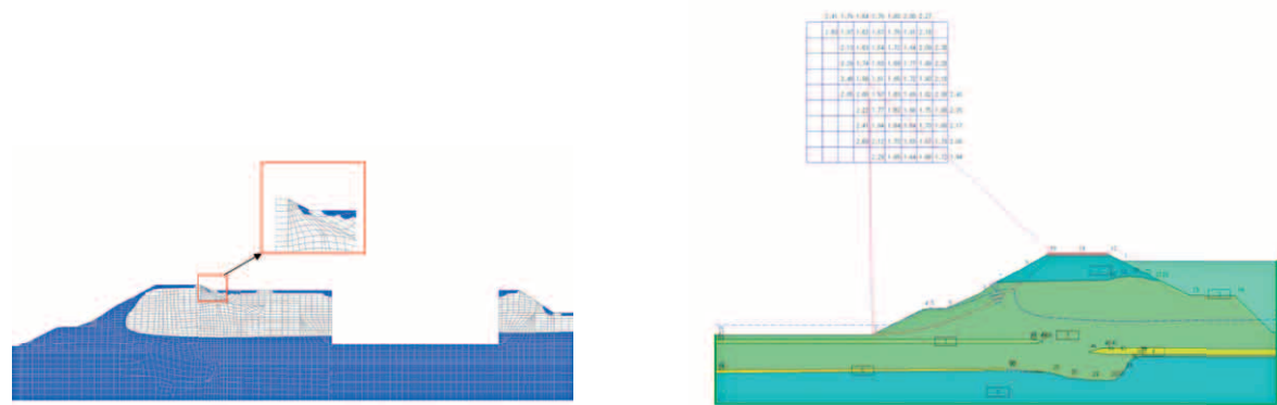
堤防の安定検討 左:浸透流解析(地下水位) 右:斜面安定解析
