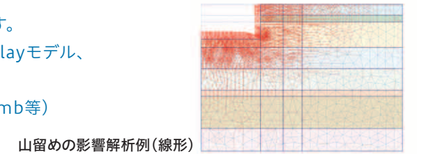
山留めの影響解析例(線形)
