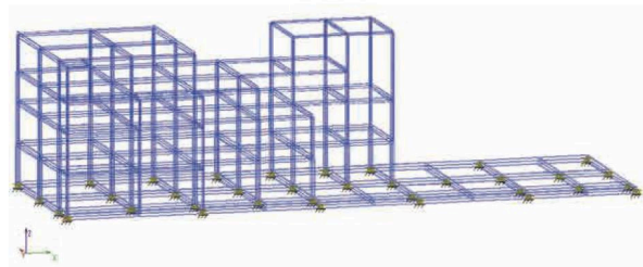
免震レトロフィット適用例
